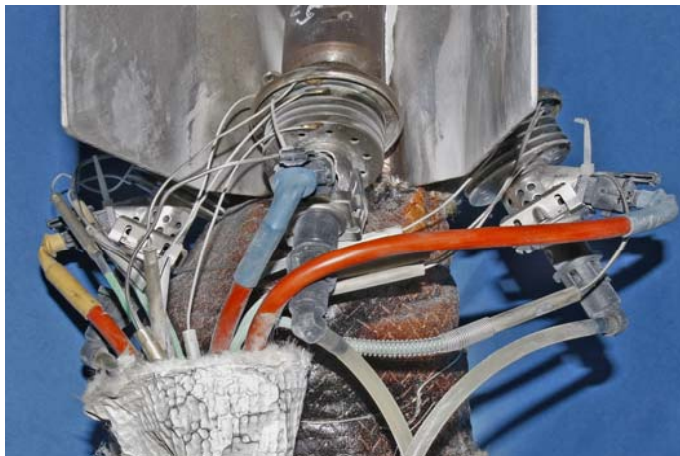
Bestückung Abgasstrang mit mehreren DeNox-Injektoren
